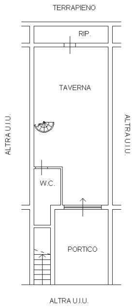
VIA DELLO SCOIATTOLO PIANTA PIANO TERRA H=2.00
