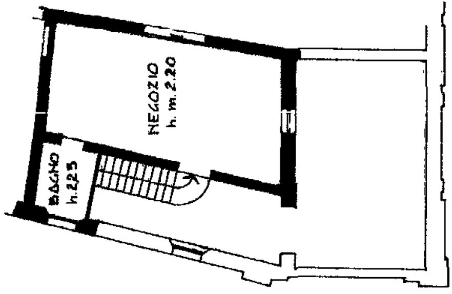
PIANO AMMEZZATO
