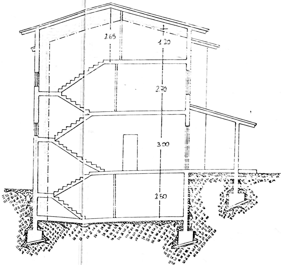
SEZIONE -
