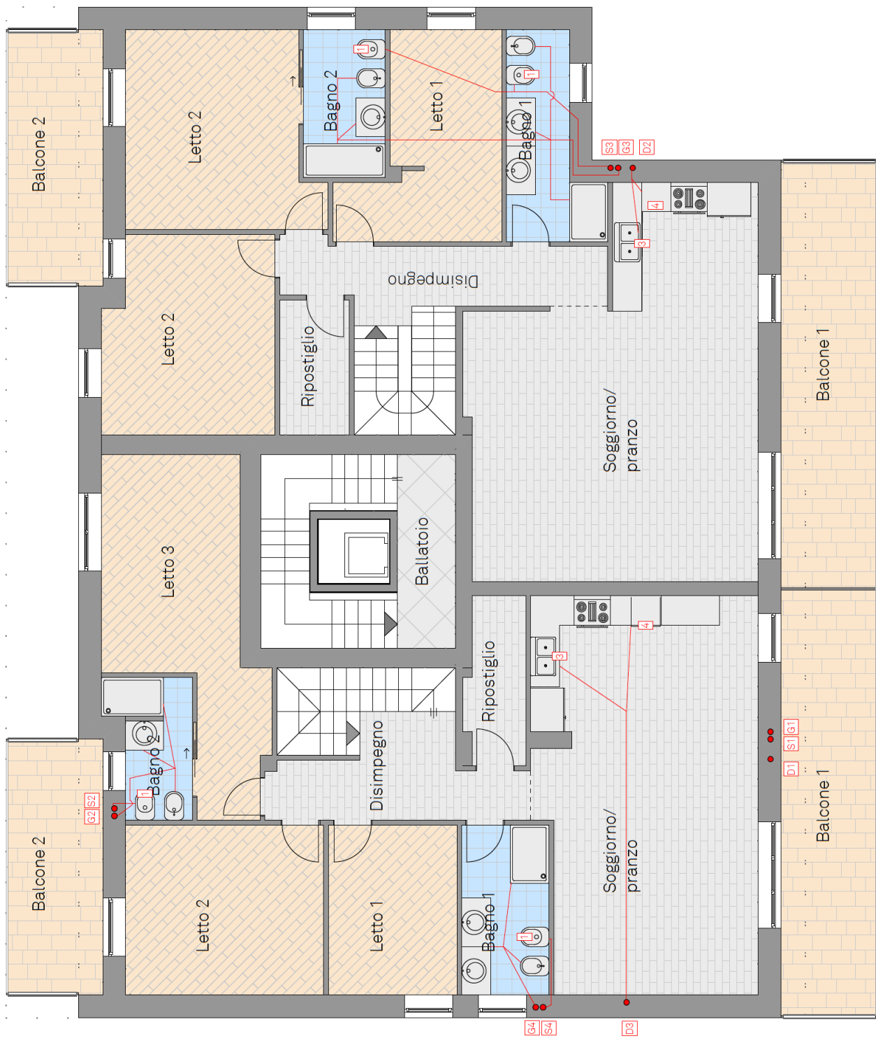
Pianta piano primo con schema fognature
